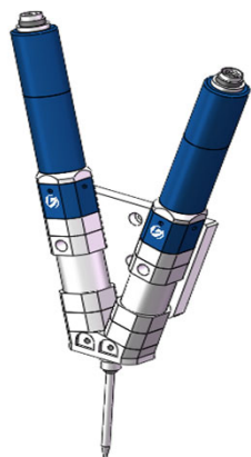
微量精密螺 杆阀 PC30
